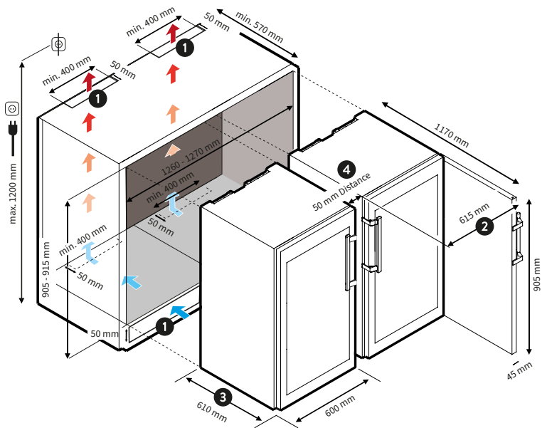
Instalación de varios dispositivos (lado a lado)
