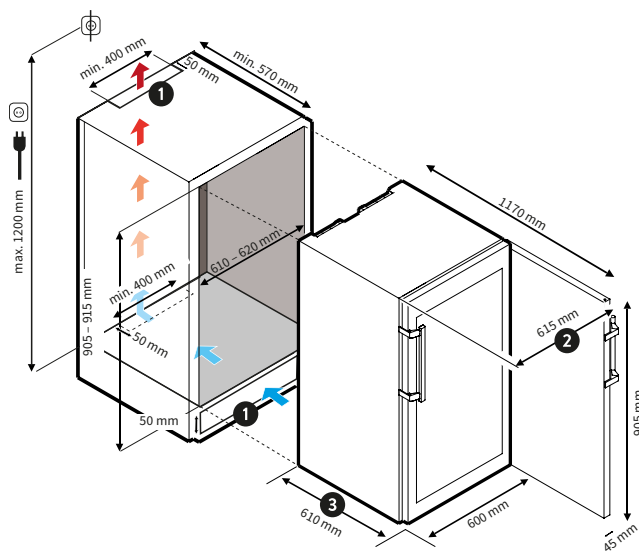
Instalación de un dispositivo
